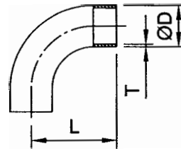
90° Long Bend
