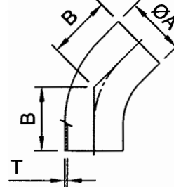
45° Long Elbow
