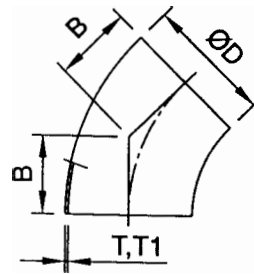
45° Elbow
