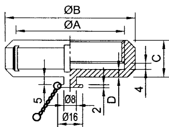
SWS Blank Nut 13RBN
