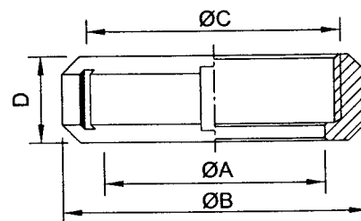
SMS Nut 6 Slots SMS-13R
