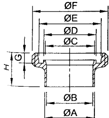
DIN Imperial Welding Male
