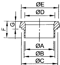
DIN Imperial Welding Liner
