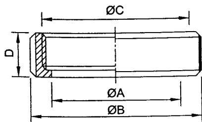
SMS-13BE Nut 4 Slots SMS-13R
