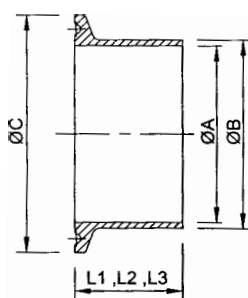
DIN Ferrule
