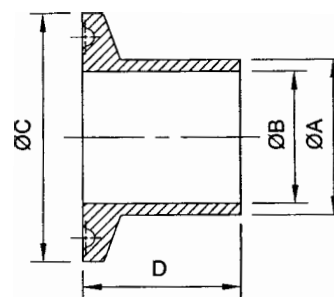
ISO Ferrule
